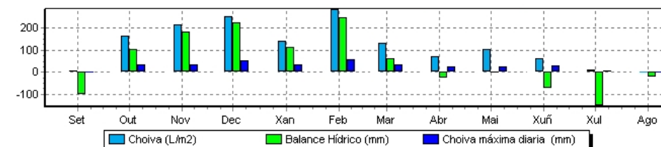
CADRO Nº 2.- VALORES DE PRECIPITACIÓN (ANO 2009)
